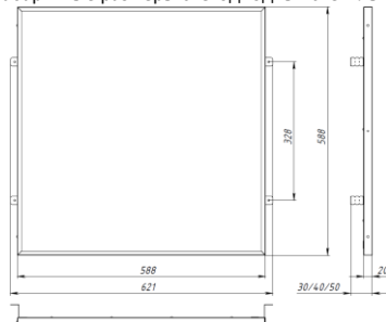
Рисунок 1 – Габаритные размеры светильника
